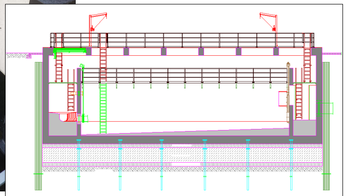
Bauwerksschnitt
