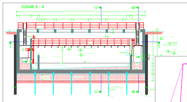
Bauwerksschnitt
