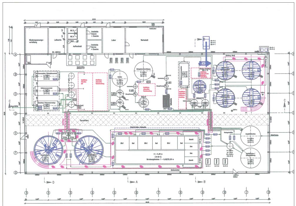
Aufstellungsplan der Demonstrations- und Prüfanlage
